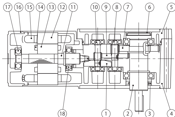
図 10-1 RNFM 形 (例：RNFM0025-03L-240)
