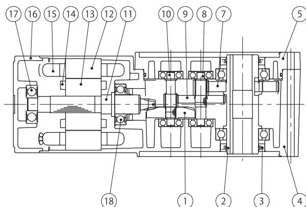
図 10-2 RNYM 形 (例：RNYM0025-03-240)
