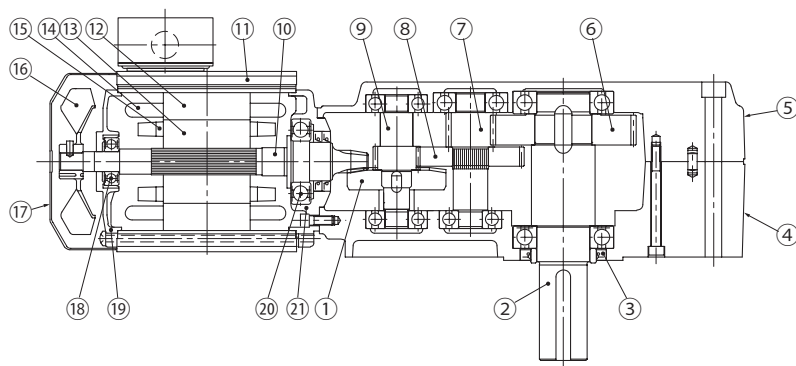
図 10-3 RNFM 形 (例 : RNFM08-50R-120)
