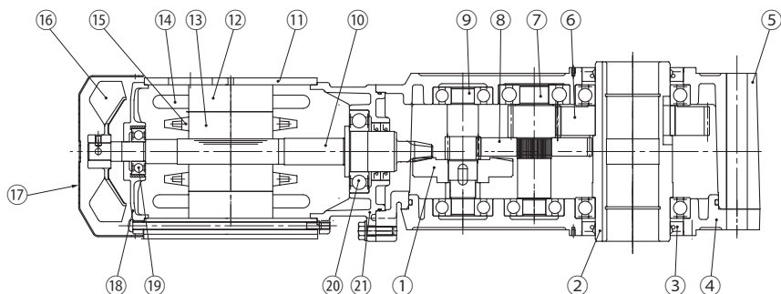
図 10-4 RNYM 形 (例 : RNYM08-1530-120)
