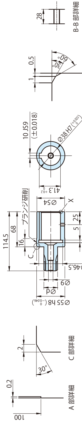
B-B部詳細
