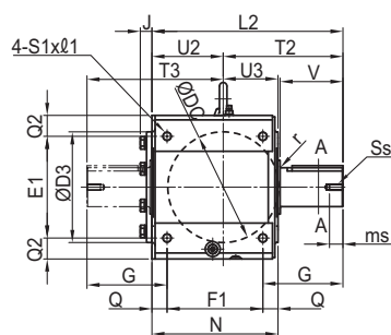
中実軸 4F18□~4F19□
