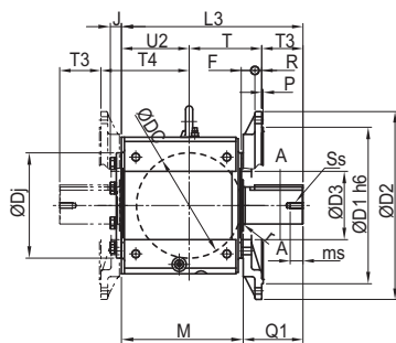
中実軸 4F18DA~4F19DB
