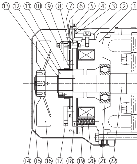
図 F42 FB-5E、FB-8E（屋内形）
