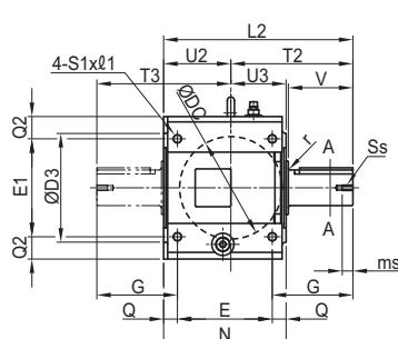
中実軸 4A10DA~4E18DB
