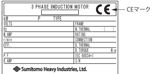
CE仕様銘板例
