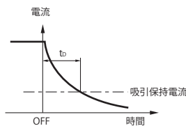
図 F34 標準回路の電流減衰カーブ
