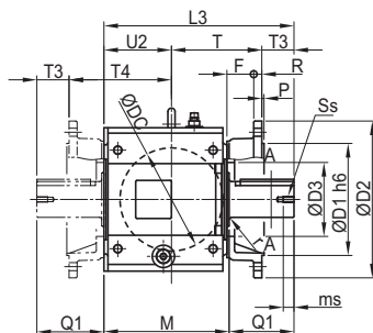
中実軸 4A10DA~4E18DB
