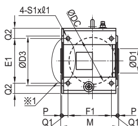
中空軸
