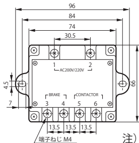
図 G22 付属整流器（直流電源装置）HD-110M3 形
