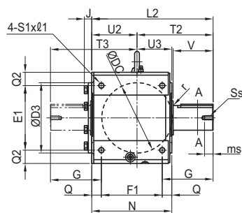
中実軸 4F18DA~4F19DB
