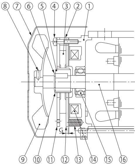
図 G8 FB-01A、FB-02A、FB-05A（屋内形） （FB-01A はファンなし）
