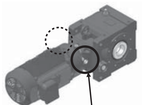
オイルゲージ逆位置 または両側取付仕様
