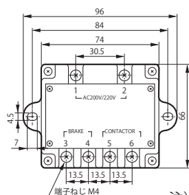
図 G37 付属整流器(直流電源装置) HD-110M3 形
