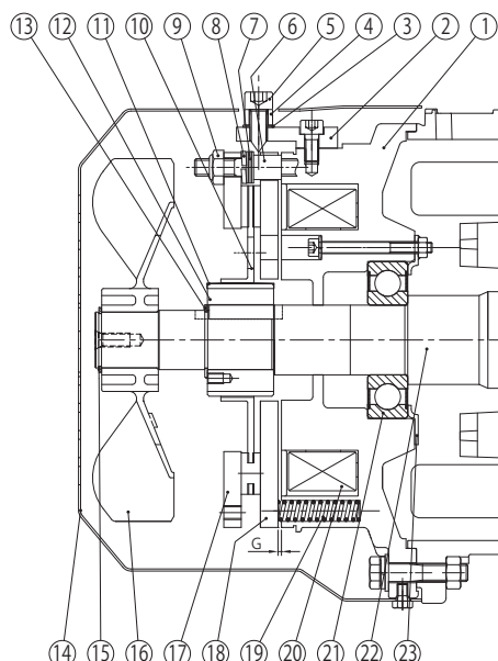
図 G18 FB-10E、FB-15E（屋内形）
