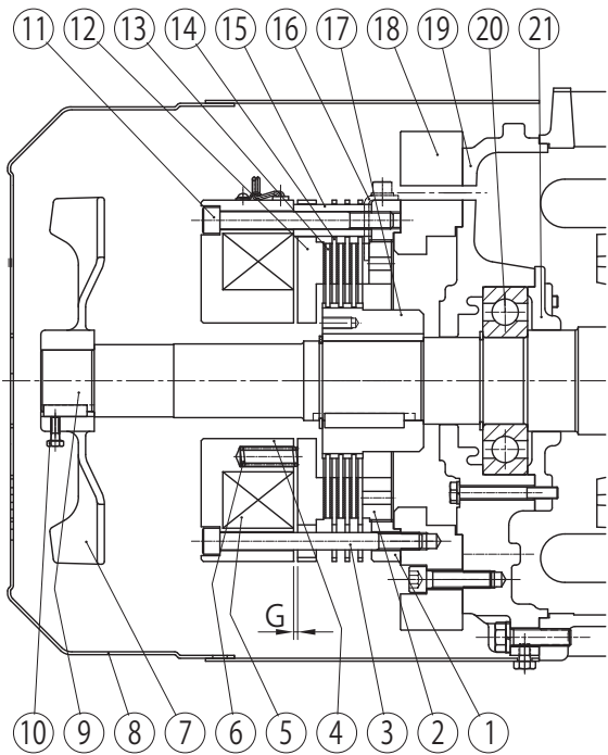
図 F46 ESB-250、ESB-250-2（屋内形）
