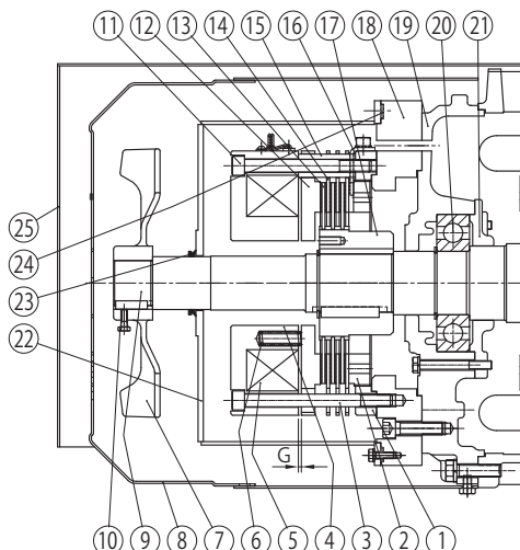
図 G36 ESB-250、ESB-250-2 (屋外形)
