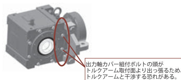
トルクアームアタッチメントタイプ取付図
