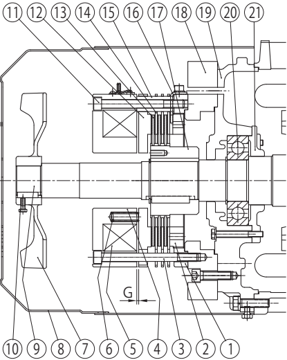
図 G21 ESB-250、ESB-250-2（屋内形）
