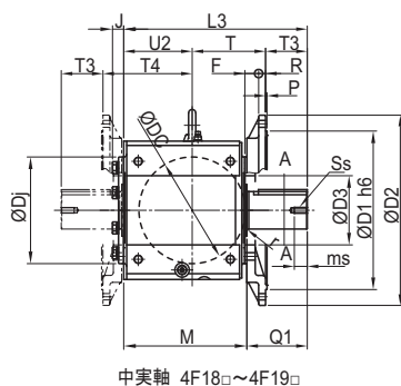
中実軸 4F18□ ~ 4F19□
