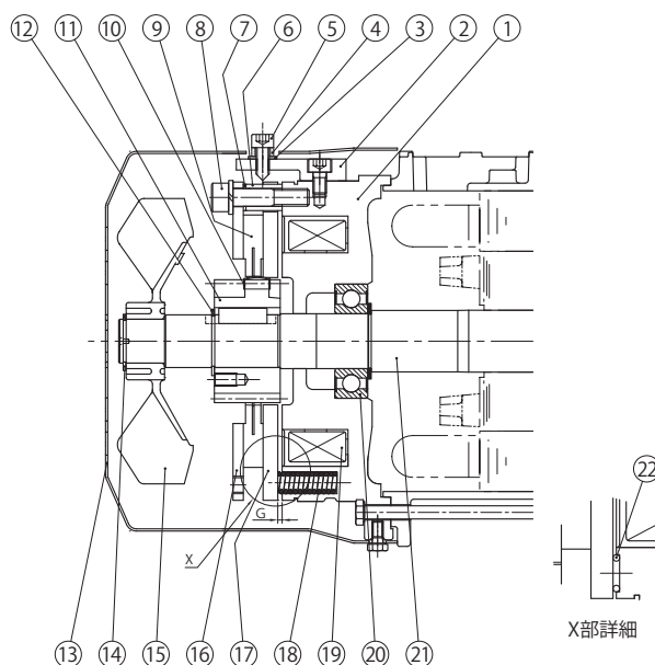
図 G11 FB-1HE、FB-2E（屋内形）
