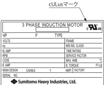
三相モータ・インバータ用 AF モータ銘板例
