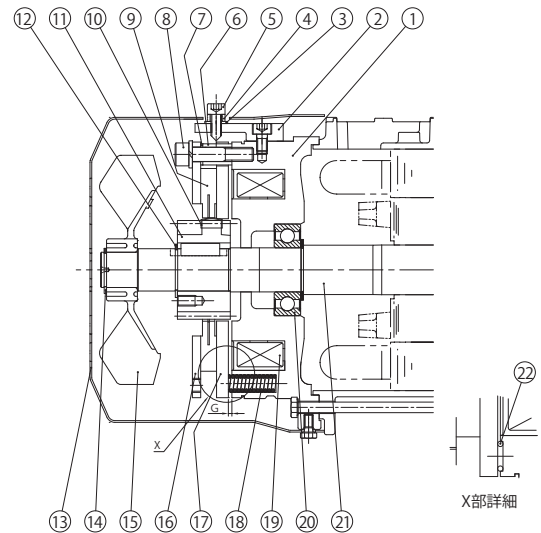
図 F40 FB-1HE、FB-2E（屋内形）
