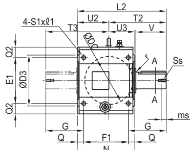
中実軸 4A10□~4E19□
