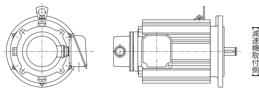
エンコーダ付モータ 製品例（モータ単体）
