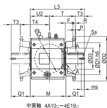
中実軸 4A10□ ~ 4E19□
