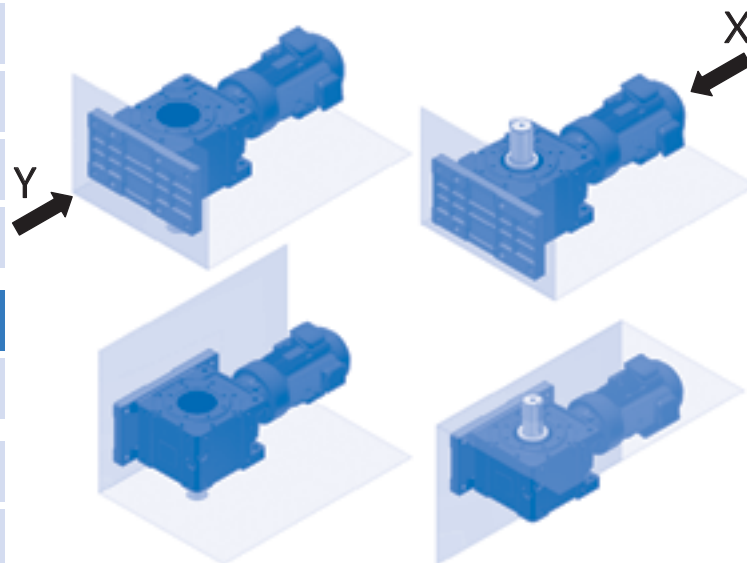
取付位置記号V5,K5
