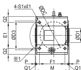
中空軸
