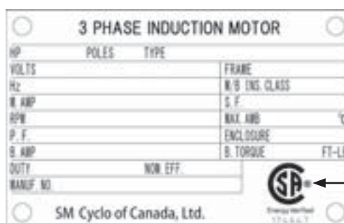
プレミアム効率三相モータ銘板例
